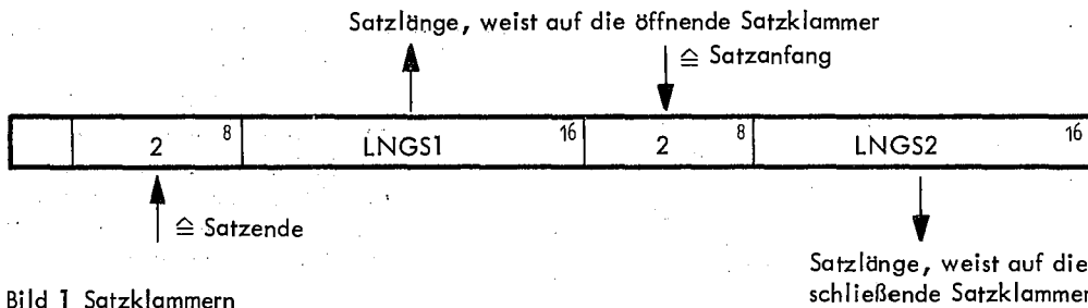
Bild 1 Satzklammern
